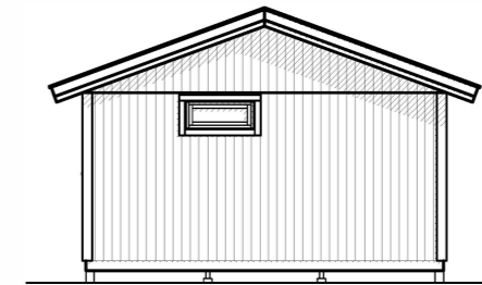
FASAD MOT
